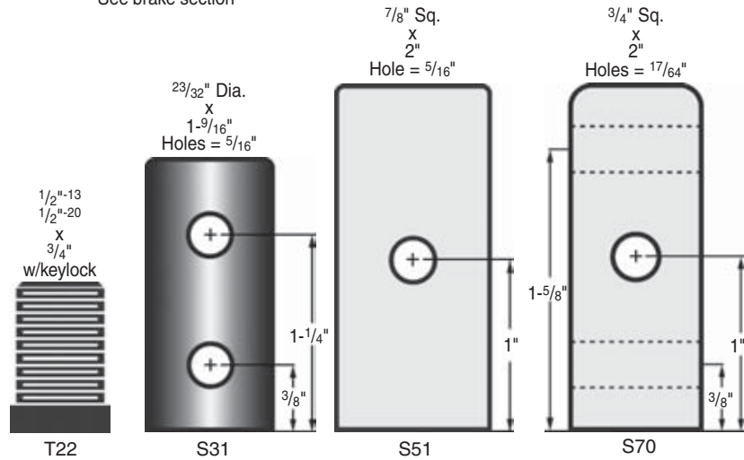
CWB Brake
